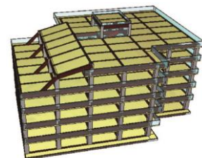
屋根に勾配、柱・梁に傾きがあるもの
